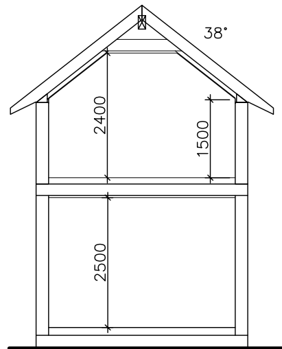
SCHNITT 2
