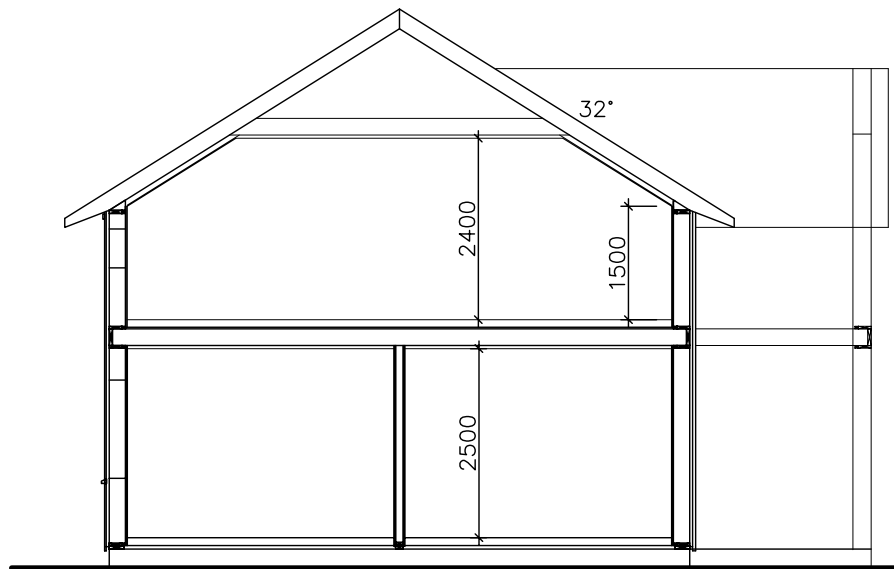
SCHNITT 1
